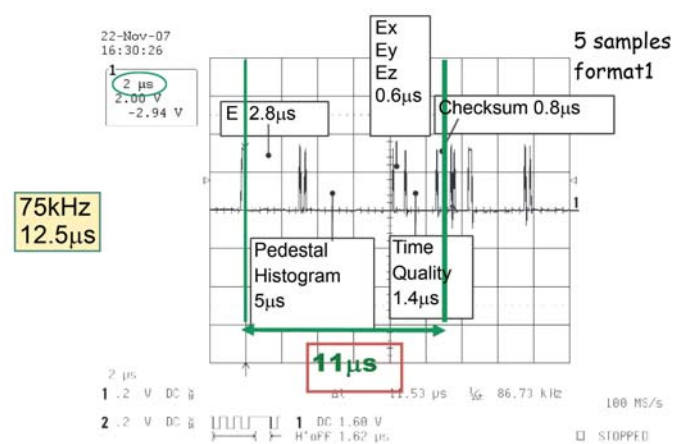
Figure 1 : Temps de calcul dans le DSP pour les étapes successives de reconstruction de l'énergie, du temps et du facteur de qualité ainsi que pour le suivi online (histogrammes de monitoring). Le temps disponible entre deux événements est au maximum de 12 µs.
