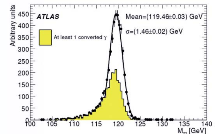
Figure 5 : Distribution de la masse invariante de paires \gamma\gamma après sélection dans des événements H \rightarrow \gamma\gamma simulés. La courbe montre tous les événements, et l'histogramme jaune les événements où au moins un des photons est converti.
