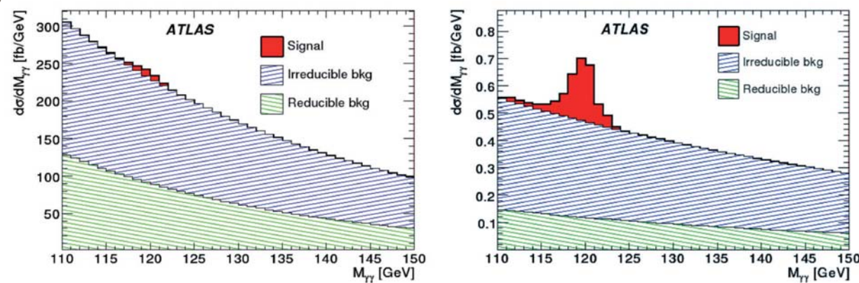
Figure 4 : Distribution de la masse invariante de paires \gamma\gamma après sélection pour des échantillons simulés de signal et bruit de fond (de haut en bas : signal, bruit de fond irréductible et réductible). La figure de gauche montre tous les événements ; celle de droite montre les événements avec deux jets associés dans la configuration attendue pour la production de Higgs par fusion de bosons de jauge intermédiaires.
