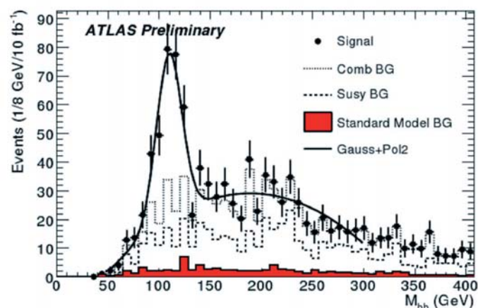
Figure 6 : Masse invariante quark antiquark b , dans le cas d'une production de Higgs dans les cascades de désintégration de particules supersymétriques dans ATLAS. Le pic du Higgs est clairement visible au dessus du bruit de fond avec une signification statistique supérieure à 10 pour 10 \text{ fb}^{-1} .
