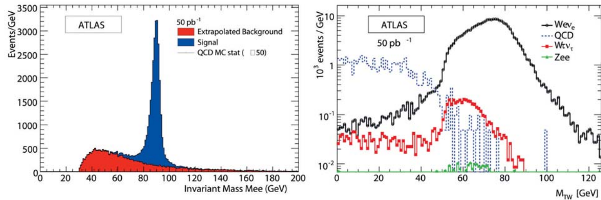
Figure 3 : La figure de gauche montre la masse invariante e^+e^- et la figure de droite la masse transverse électron-neutrino.
