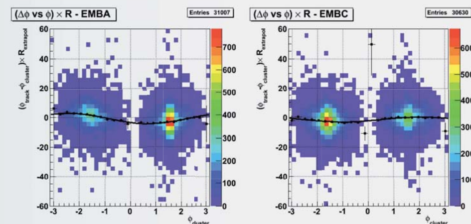
Figure 2 : L'imperfection d'alignement du détecteur électromagnétique tonneau crée une dépendance sinusoïdale sur la différence de position en phi entre les traces du trajectomètre et les amas calorimétriques. L'amplitude de cette sinusoïde est proportionnelle à la différence d'alignement.
